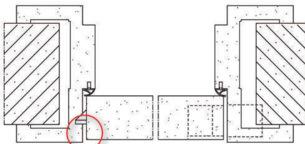
Stumpf einschlagendes Element, EE Zarge
